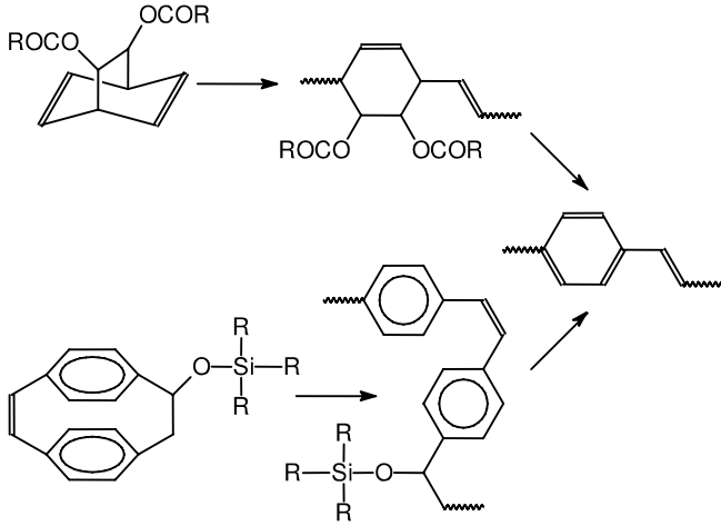
الشكل (3-5) : اصطناع PPV بواسطة البلمرة بالمنافلة الفاتحة للحلقات 11,12
